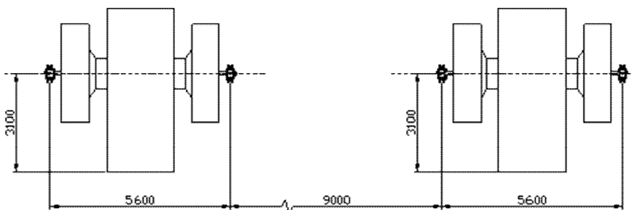
Rys. 1. Schemat rozmieszczenia łożysk badanego wentylatora.
